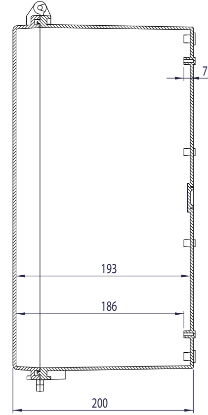
KESIT A-A
