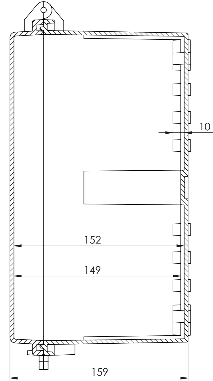
KESİT A-A
