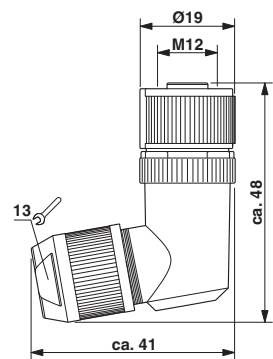
Dessin coté
