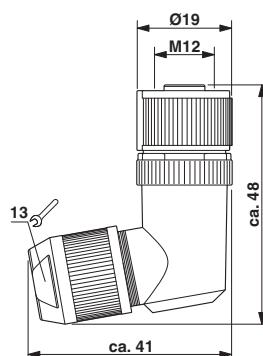
Dessin coté
