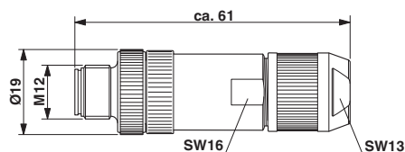
Dessin coté
