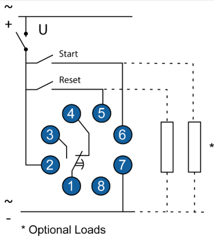
MDF1
