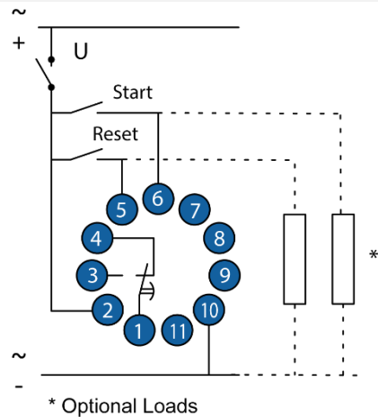
GDF1
