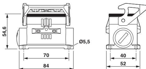
Dessin coté
