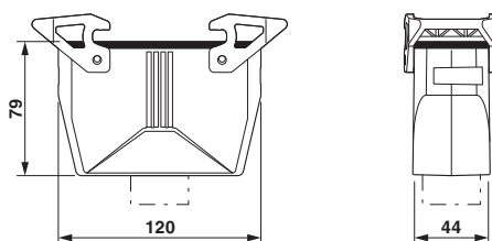
Dessin coté
