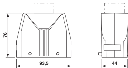
Dessin coté
