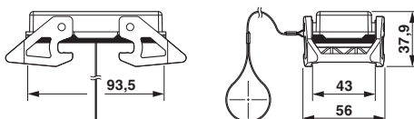
Dessin coté
