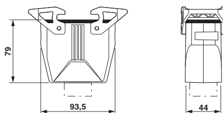
Dessin coté
