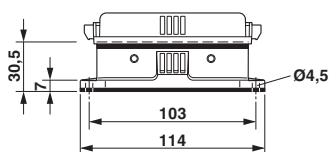
Dessin coté
