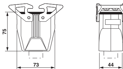
Dessin coté
