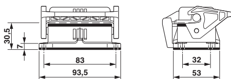
Dessin coté
