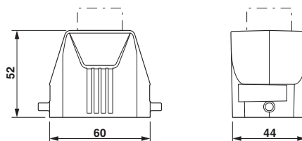
Dessin coté
