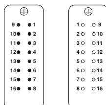
Schéma des pôles côté câblage
