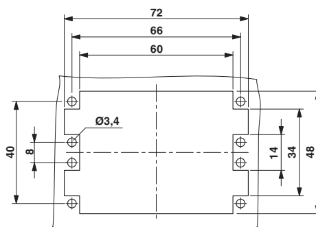
Dessin coté
