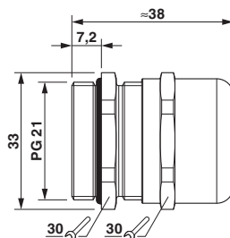
Dessin coté
