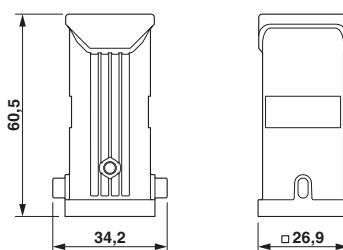
Dessin coté
