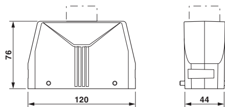
Dessin coté
