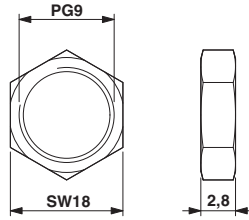
Dessin coté
