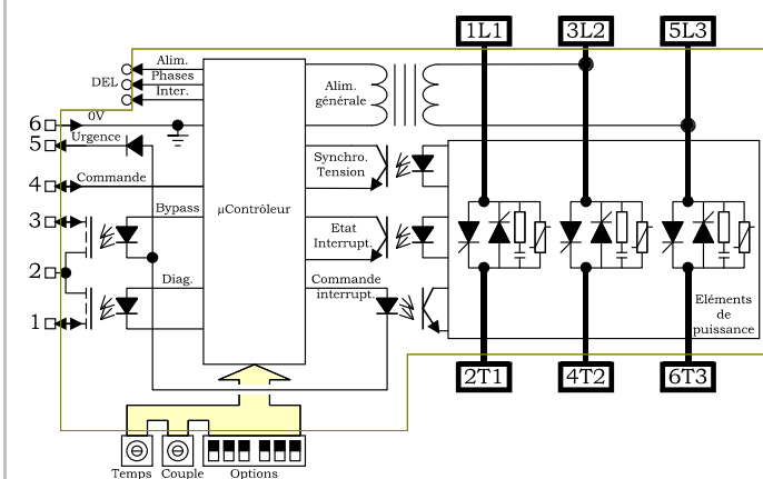
Fig. 1 SYNOPTIQUE INTERNE
