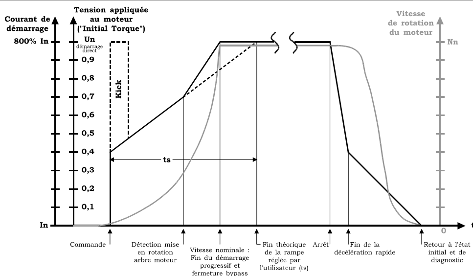
Fig. 3 DESCRIPTION DES DIFFERENTS PARAMETRES DE REGLAGE POUR LE DEMARRAGE
