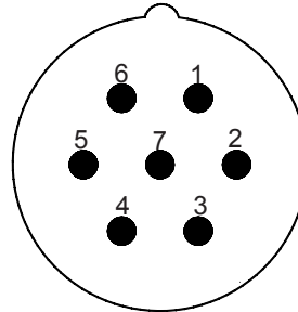
Mâle - Male - Stift
