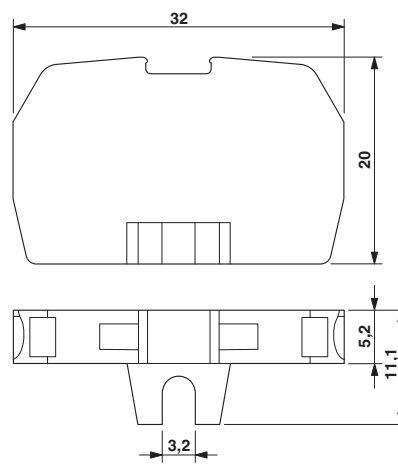
Dessin coté
