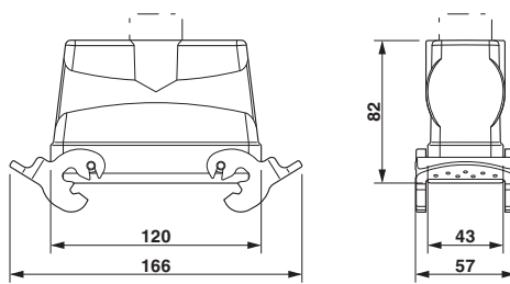
Dessin coté
