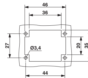
Dessin coté
