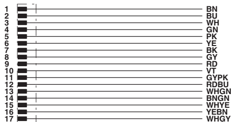
Schéma électrique
