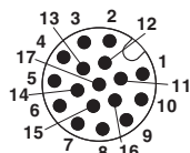
Dessin schématique
