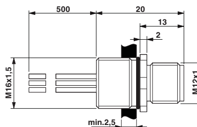
Dessin coté
