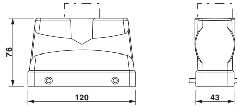
Dessin coté
