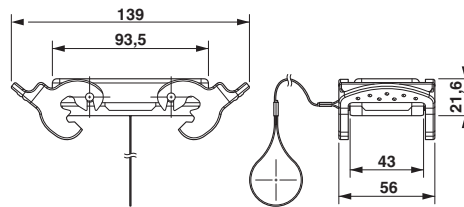
Dessin coté
