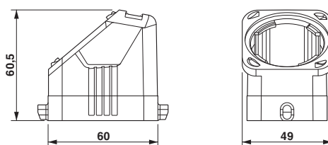
Dessin coté
