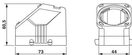
Dessin coté
