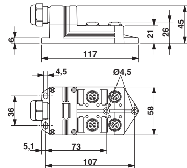
Dessin coté
