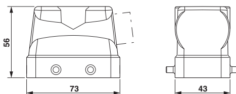
Dessin coté
