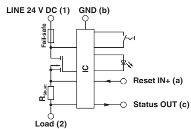
Schéma électrique
