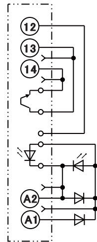
12 Vc.c. Disposition des bornes / connexions internes (vue de dessus)
