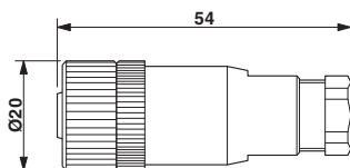
Connecteur femelle M12 x 1, droit
