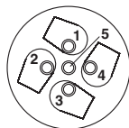
Côté connexion câble M12 (connexion vissée)
