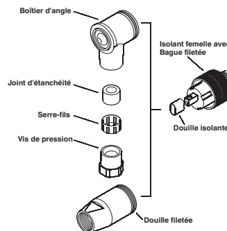
Connecteur mâle/femelle M12
