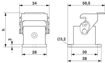
Dessin coté
