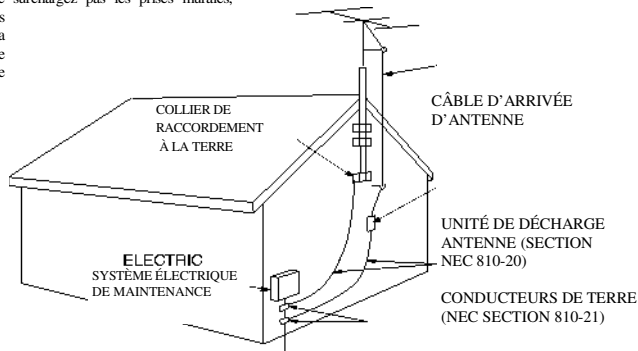
SYSTÈME ÉLECTRIQUE D'ÉLECTRODES RELIÉ À LA TERRE (NEC ART 250, PIÈCE
