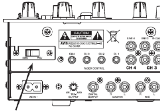
Commutateur de sélection de voltage
