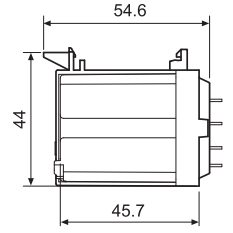
062.08 avec relais monté
