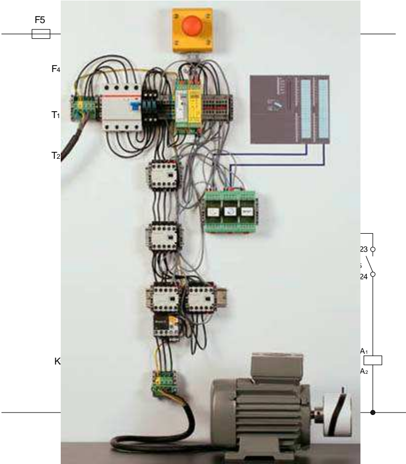
Câblage classique
