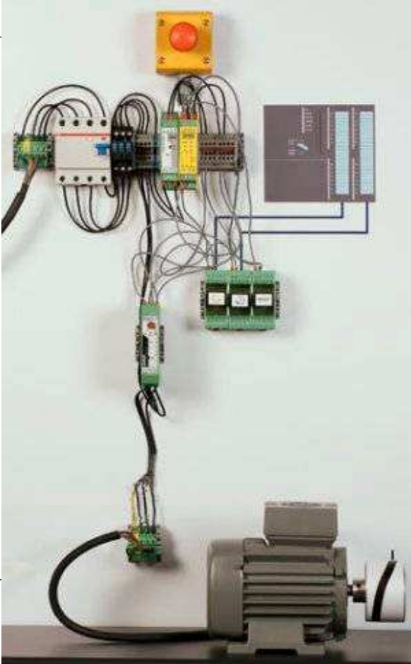
Câblage Contactron
