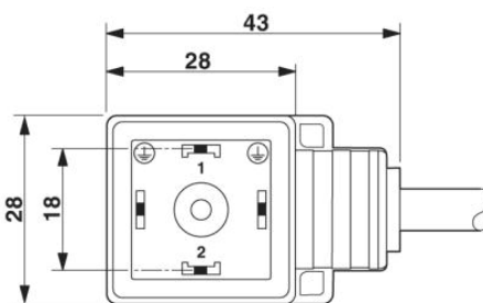
Connecteur pour électrovanne, type A Connecteur pour électrovanne, type A, vue latérale
