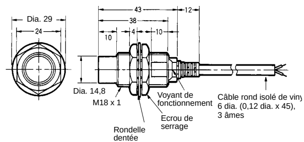
Fig. 8 : E2EG-X18MC□/B□
