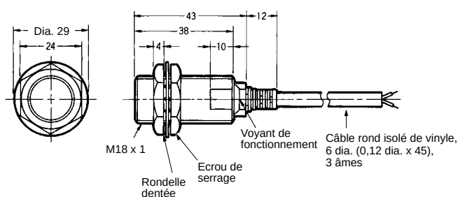
Fig. 7 : E2EG-X10C□/B□
