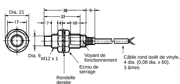
Fig. 6 : E2EG-X10MC□/B□
