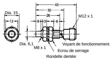
Fig. 10 : E2EG-X2MC□-M1/B□-M1
