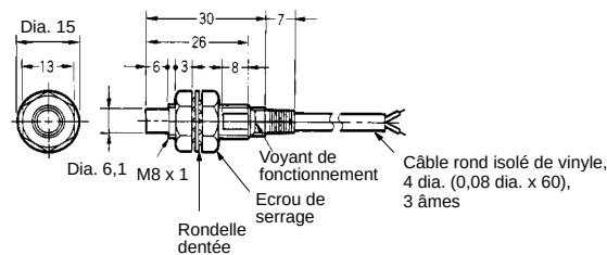
Fig. 2 : E2EG-X2MC□/B□
