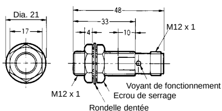
Fig. 11 : E2EG-X2C□-M1/B□-M1
