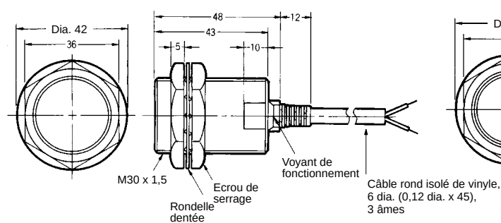
Fig. 7 : E2EG-X10C□/B□
