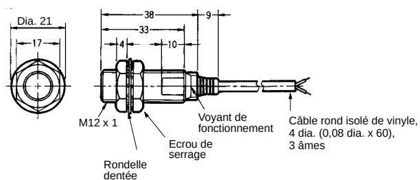
Fig. 3 : E2EG-X2C□/B□
