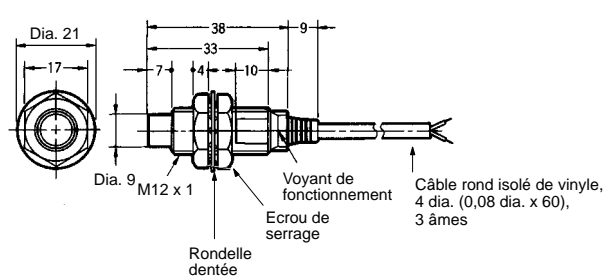
Fig. 6 : E2EG-X10MC□/B□
