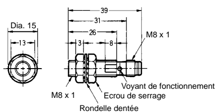
Fig. 17 : E2EG-X1R5C1-M3/B1-M3
