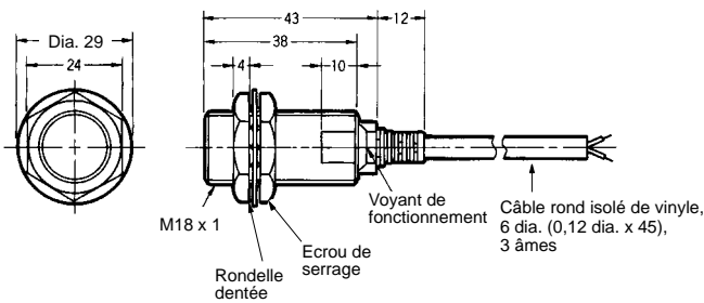
Fig. 7 : E2EG-X10C□/B□
