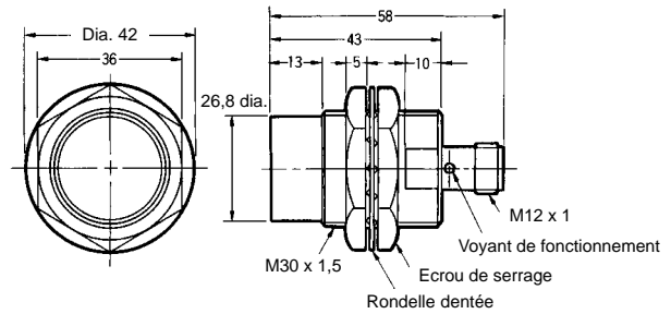
Fig. 16 : E2EG-X18MC□-M1/B□-M1
