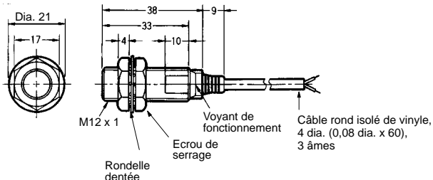
Fig. 3 : E2EG-X2C□/B□
