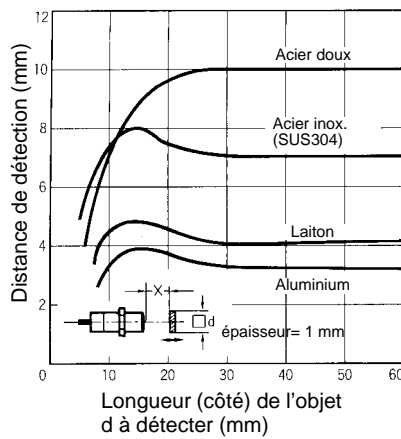
E2EG-X10MC□/B□
