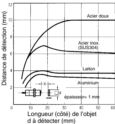
E2EG-X10MC□/B□
