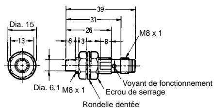
Fig. 18 : E2EG-X2MC1-M3/B1-M3
