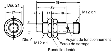
Fig. 12 : E2EG-X5MC□-M1/B□-M1
