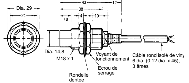
Fig. 8 : E2EG-X18MC□/B□
