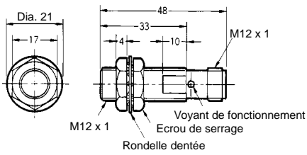
Fig. 11 : E2EG-X2C□-M1/B□-M1
