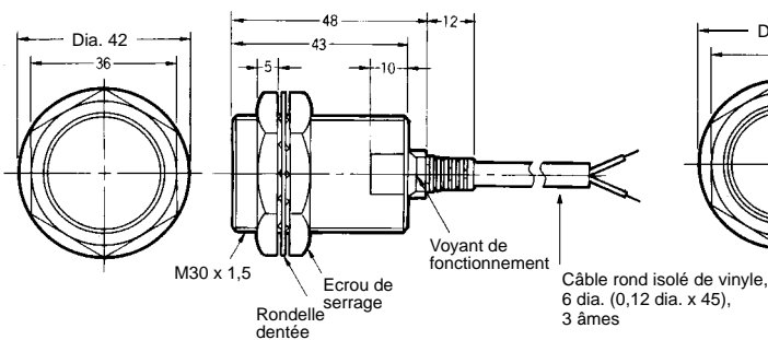
Fig. 7 : E2EG-X10C□/B□
