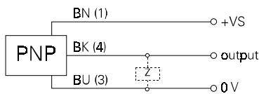
Anschlussbelegung
