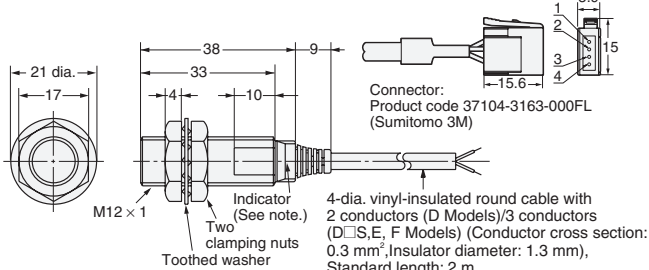
Fig. 8 : E2E-X3D□-N E2E-X2E□/F□
