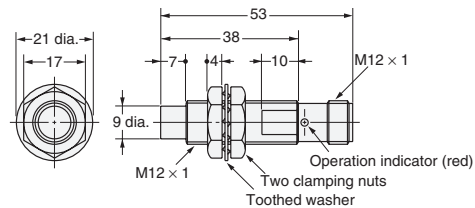
Fig. 24 : E2E-X14MD□-M1(G)/E2E-X10ME□-M1/F□-M1 E2E-X10MY□-M1
