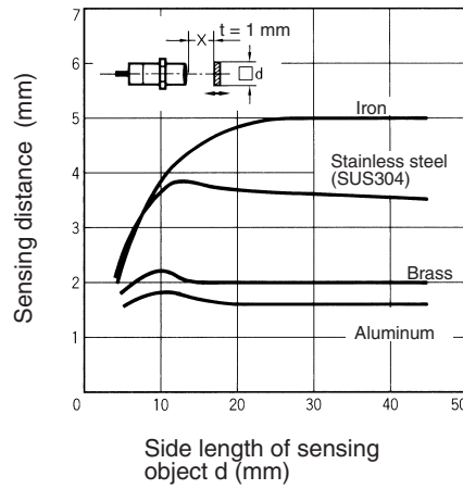
E2E-X5ME□/F□ E2E-X5MY□
