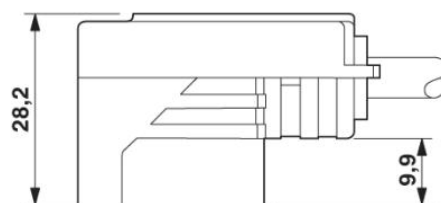
Connecteur pour électrovanne, type B, vue latérale
