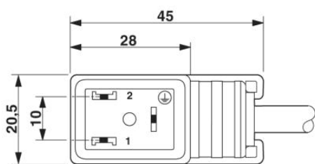
Connecteur pour électrovanne, type B
