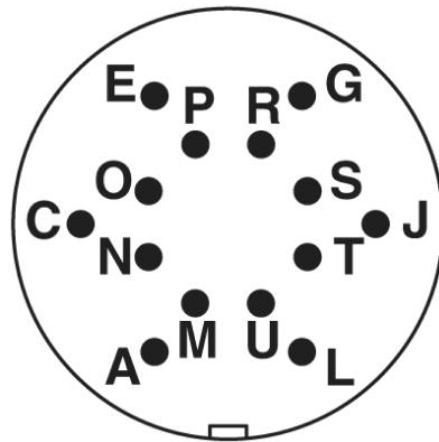
Raccordement enfichable M16 mâle; 14 pôles
