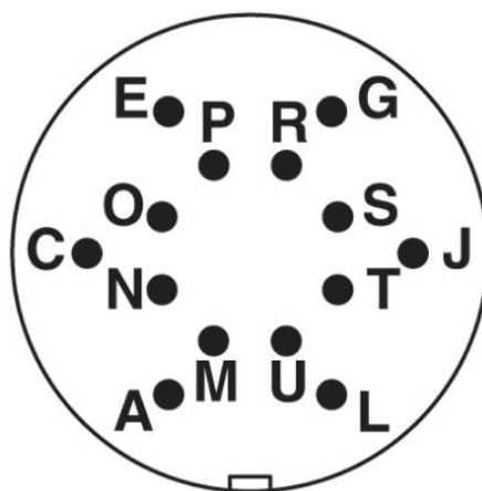
Schéma des pôles raccord enfichable M16, 14 pôles
