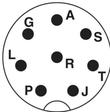
Raccordement enfichable M12 mâle; 8 pôles
