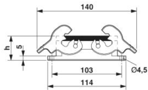
Dessin coté
