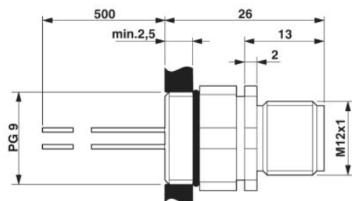
Connecteur mâle à encastrer M12, positionnable
